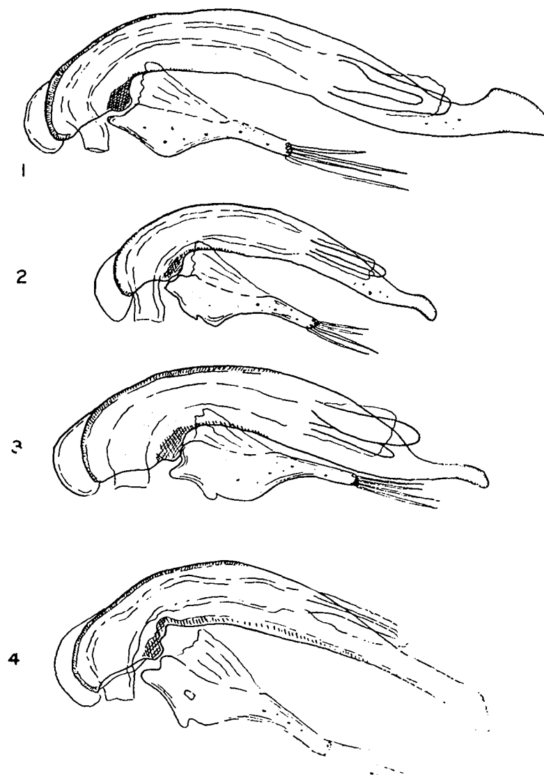
FIGURE 4. Aedeagi of Pseudanophthalmus . (1) P. templetoni vanburensis n. subsp., paratype, X62. (2) P. robustus megosteus n. subsp., paratype, Big Bone Cave, X62. (3) P. robustus farrelli n. subsp., holotype X62. (4) P. robustus lupus n. subsp., paratype, X82.
